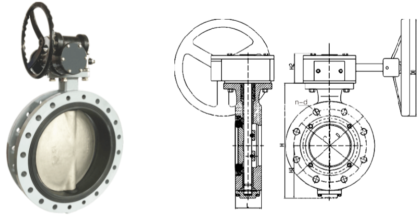
设计标准 Valve design
